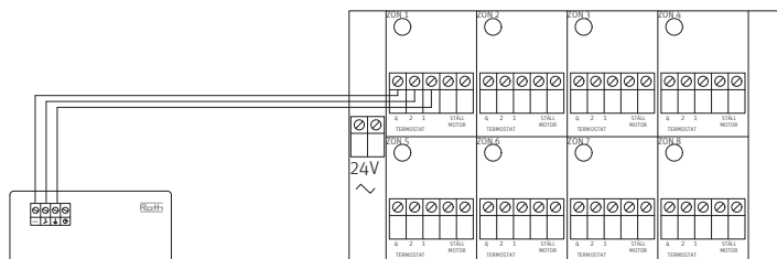
Kopplingsplint RSK nr: 242 10 15
