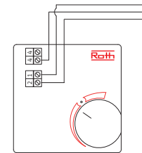
Rumstermostat elektronisk RSK nr: 242 10 13
