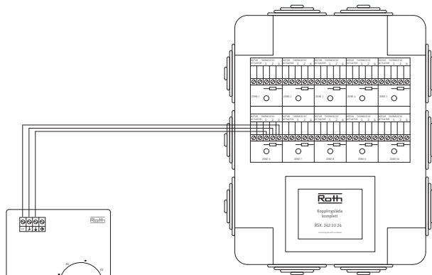
Kopplingslåda komplett RSK nr: 242 10 24
