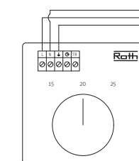
CABLE rumstermostat RSK nr: 242 24 59
